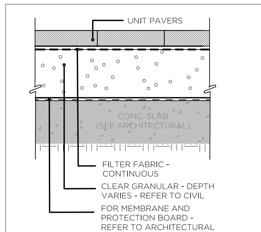
5 UNIT PAVERS ON SLAB N.T.S. L-02
