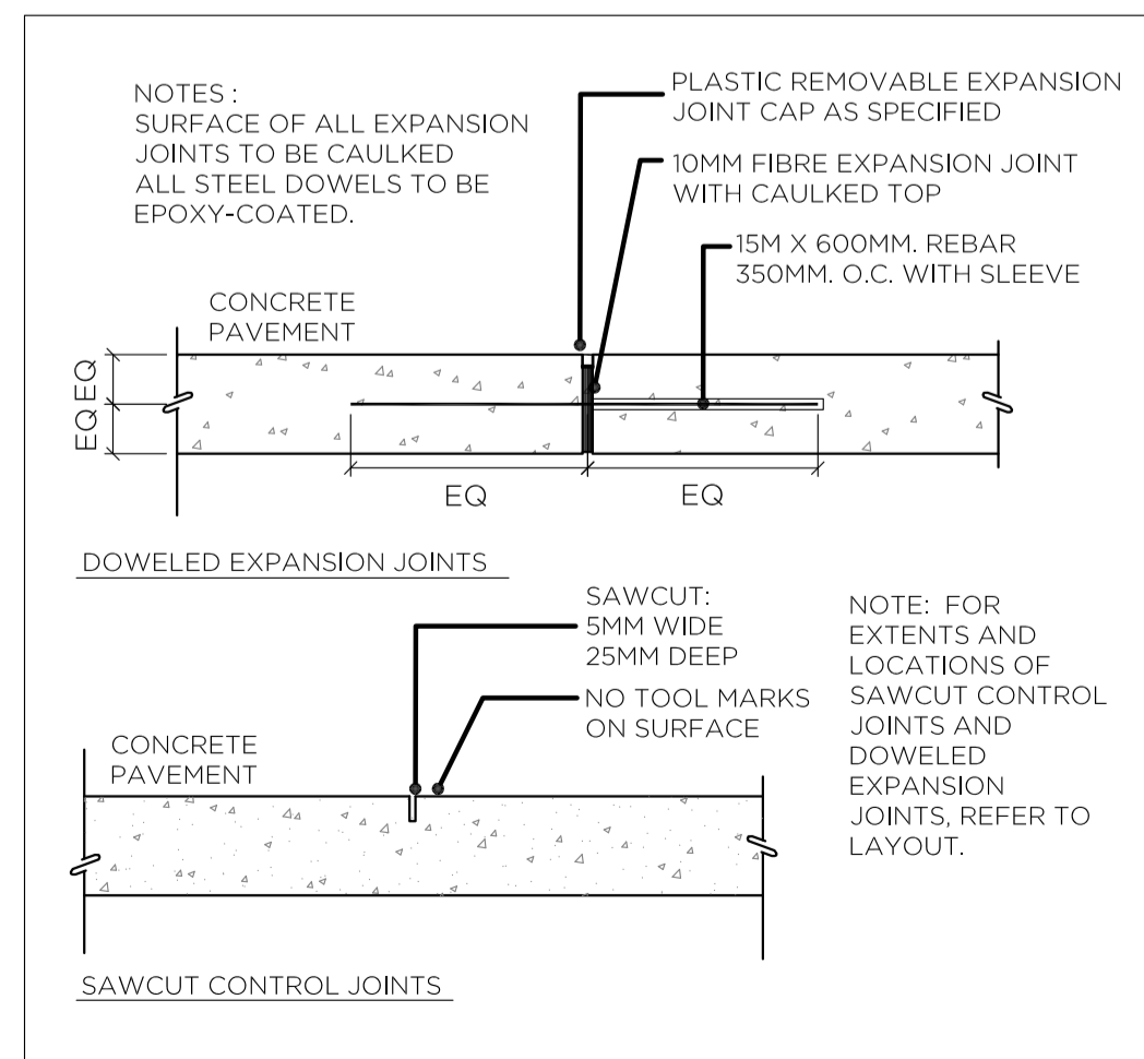
7 CONCRETE JOINTING N.T.S. L-01
