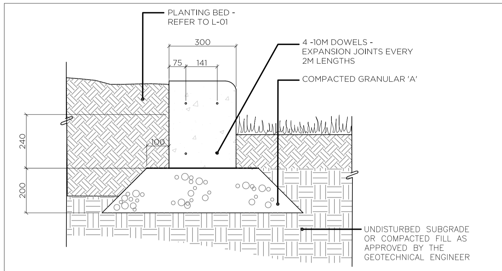
2 LANDSCAPE CURB N.T.S. L-02
