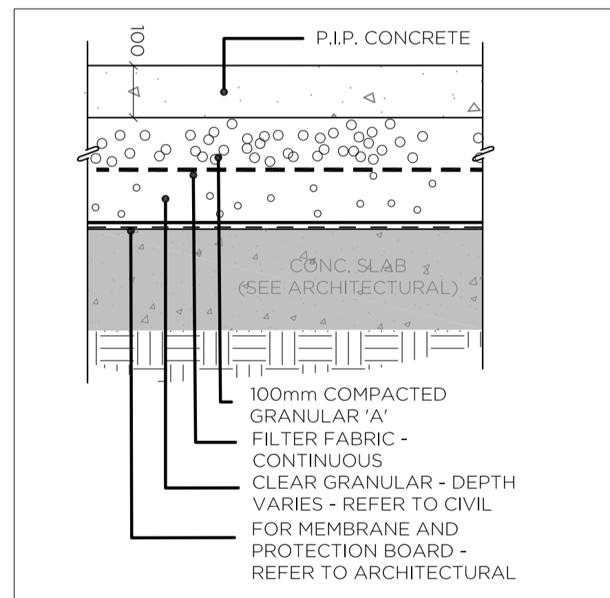
4 CONCRETE PAVEMENT ON SLAB N.T.S. L-02
