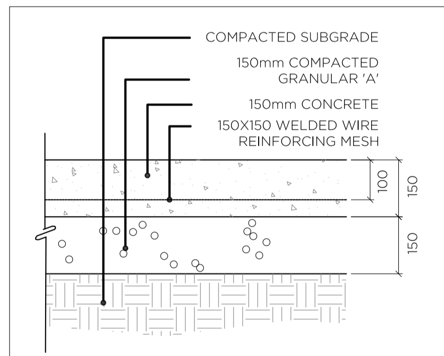
3 CONCRETE PAVEMENT N.T.S. L-02
