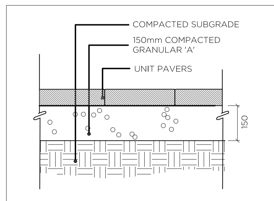
6 UNIT PAVERS N.T.S. L-02
