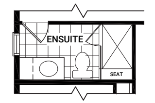
OPTIONAL ENSUITE 4 FT SHOWER PLUS BENCH
