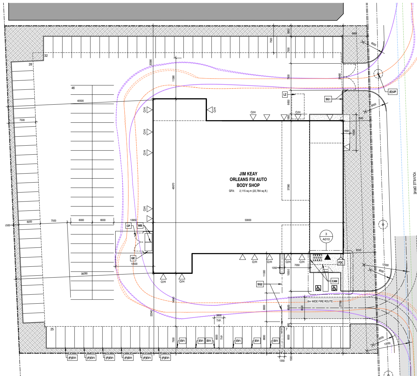
2 SITE PLAN A010 SCALE: 1 : 300
