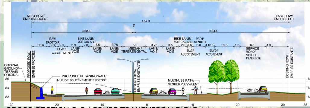
CROSS-SECTION G-G / COUPE TRANSVERSALE G-G
