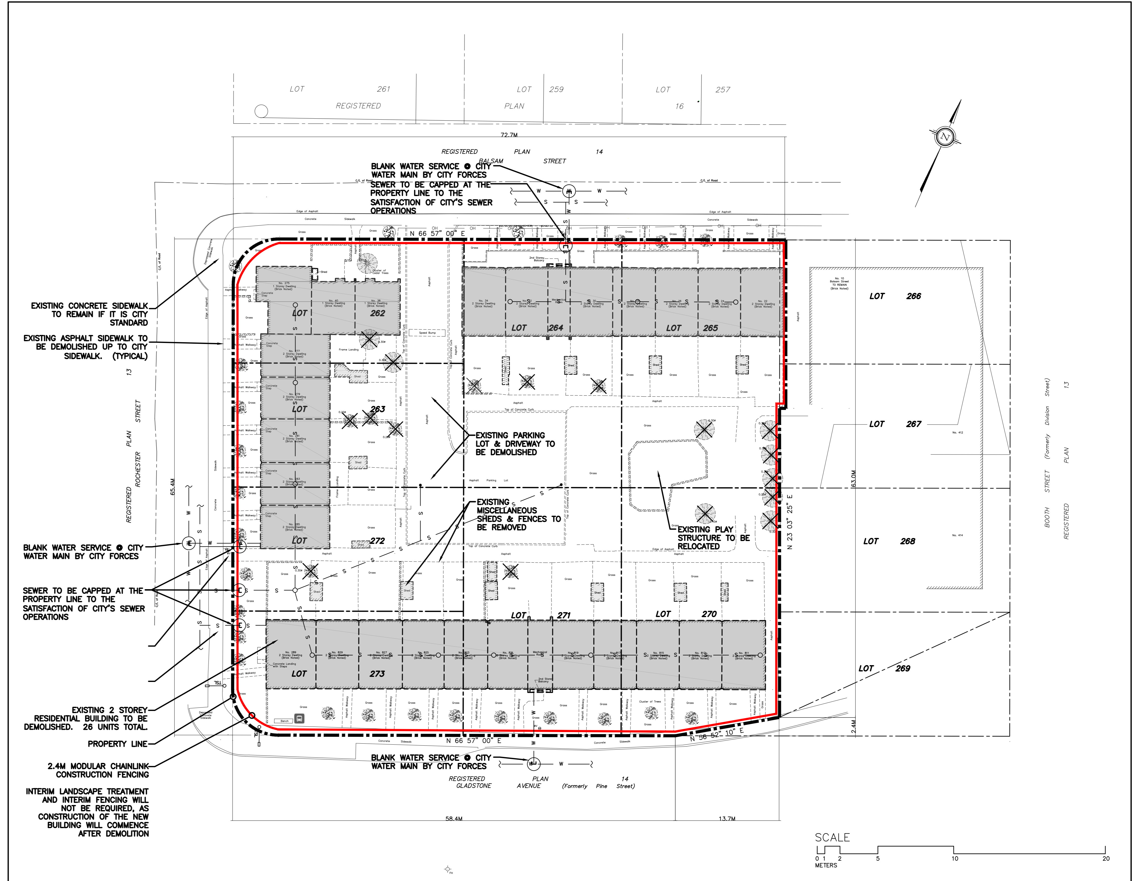
2 DEMOLITION PLAN A-1 1 : 250
