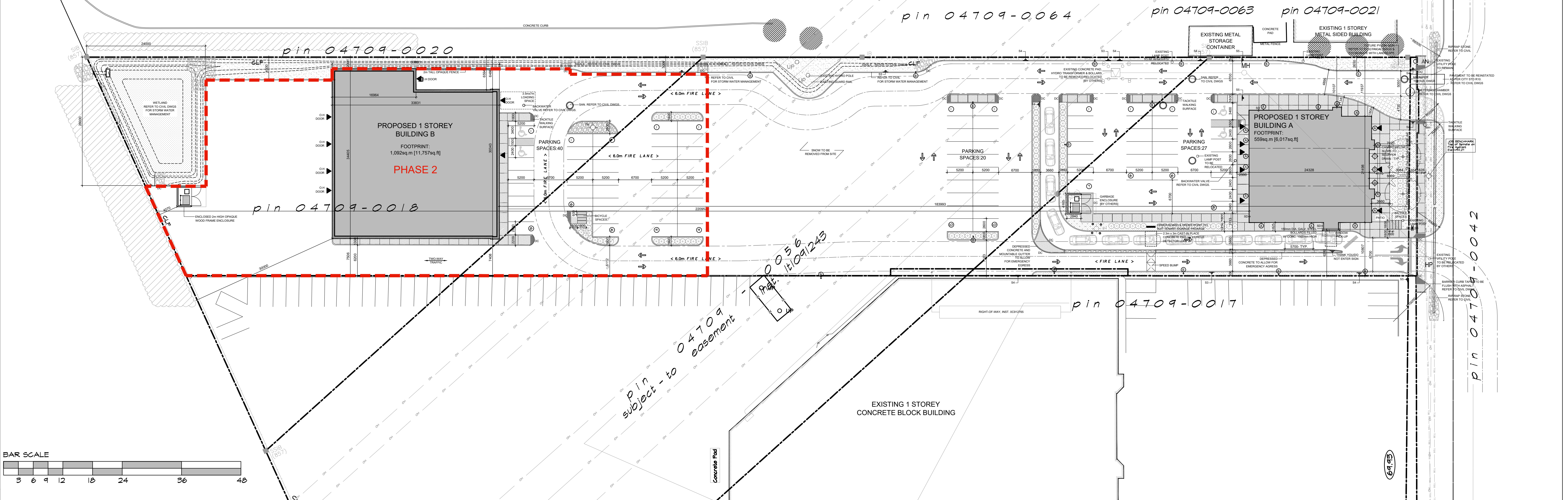
01 SITE PLAN SCALE: 1:400
