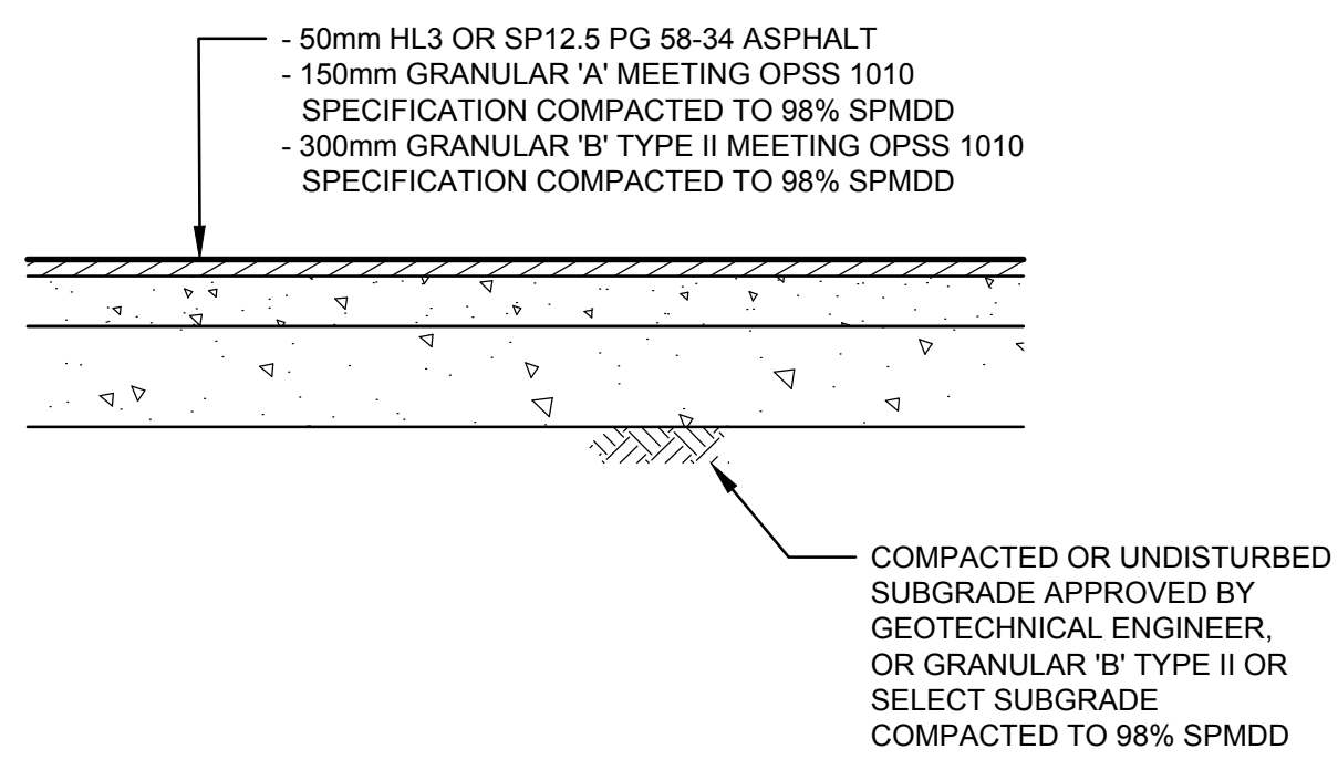
LIGHT DUTY PAVEMENT N.T.S.
