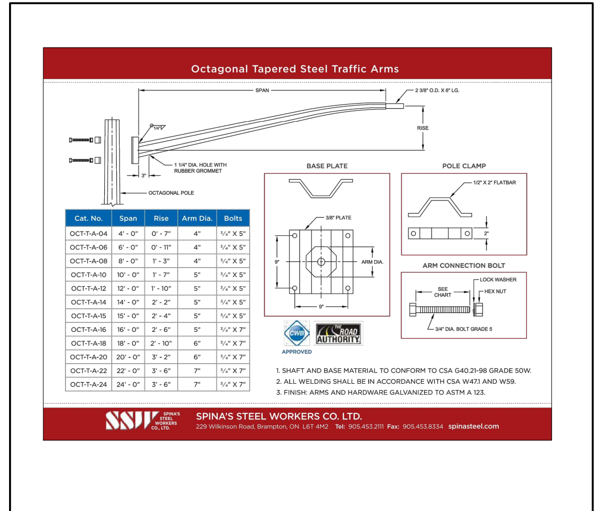
4 TAPERED STEEL STEEL TRAFFIC ARMS SCALE: N.T.S.
