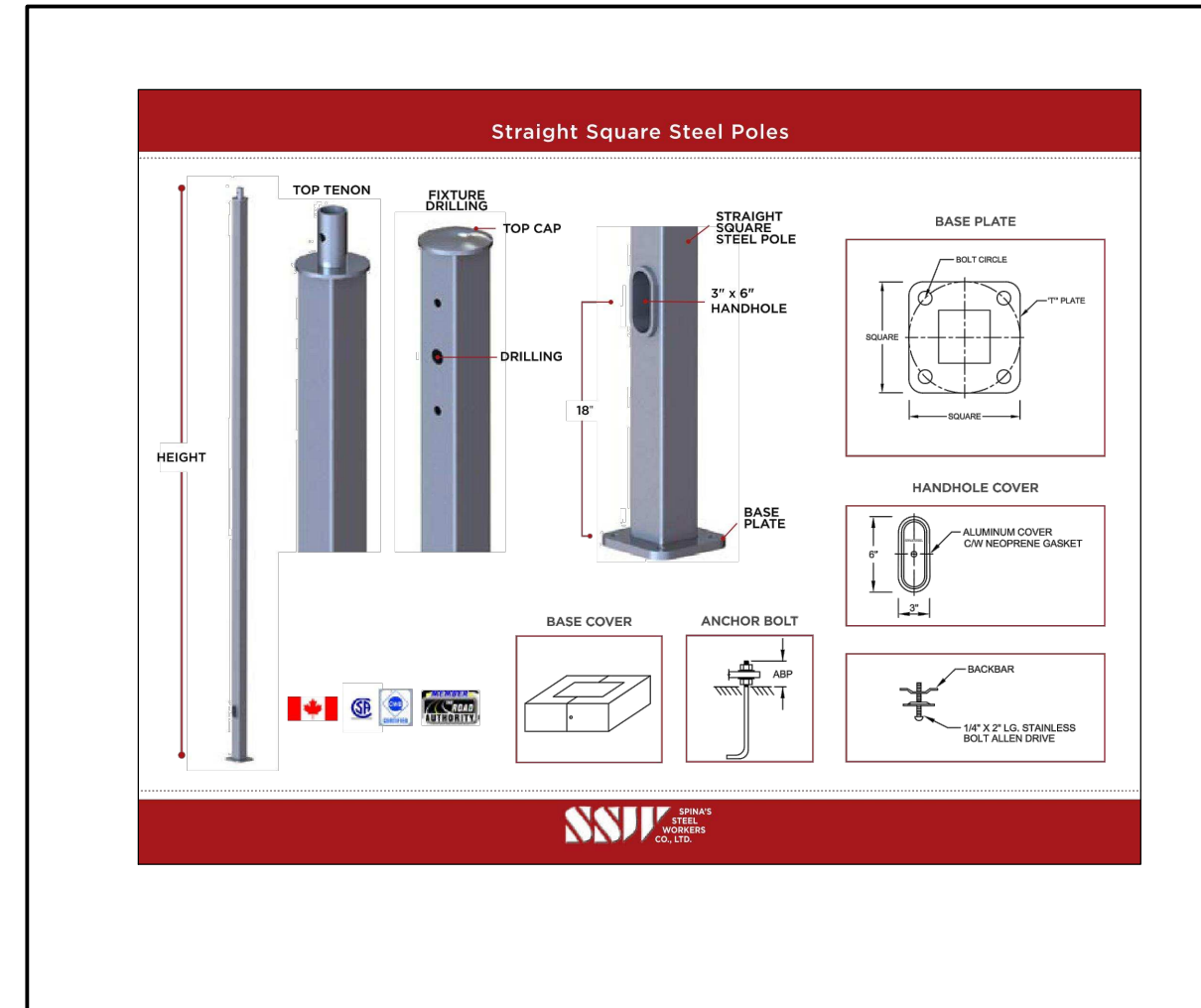
3 SQUARE STREET POLES SCALE: N.T.S.
