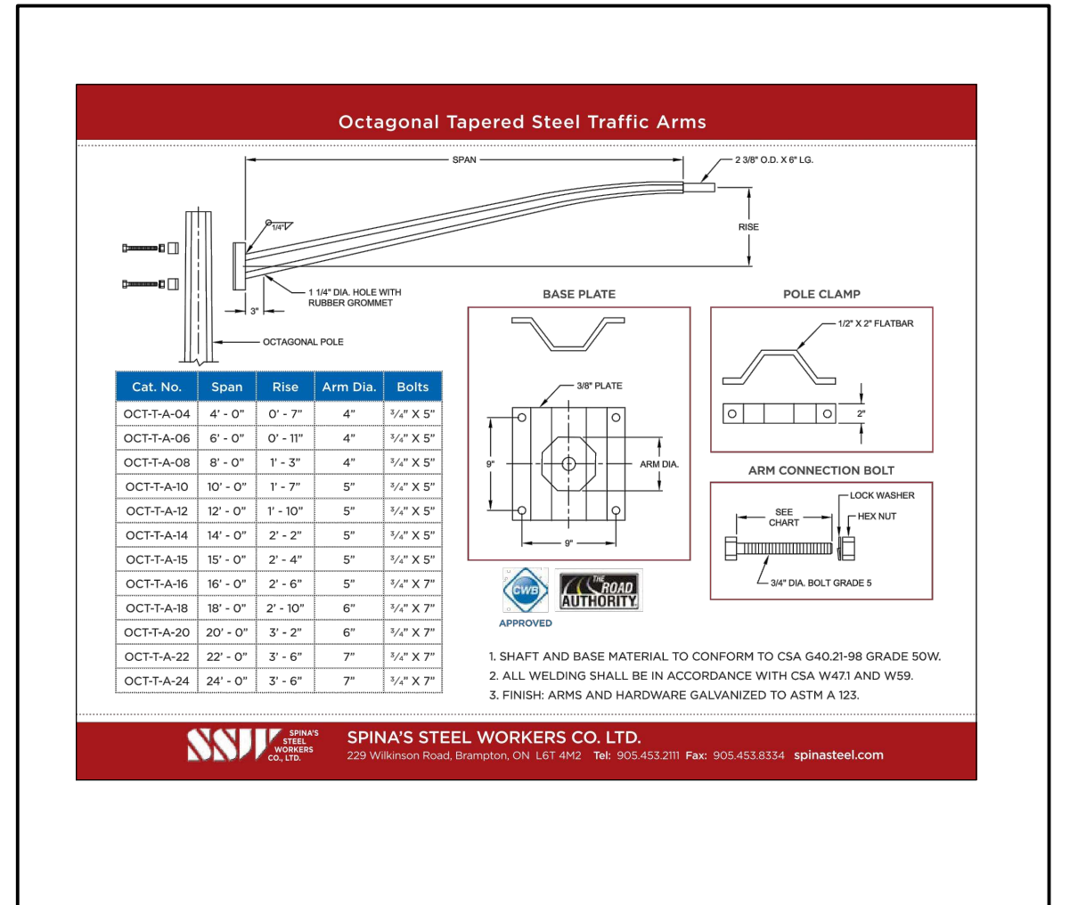
4 TAPERED STEEL TRAFFIC ARMS SCALE: N.T.S.
