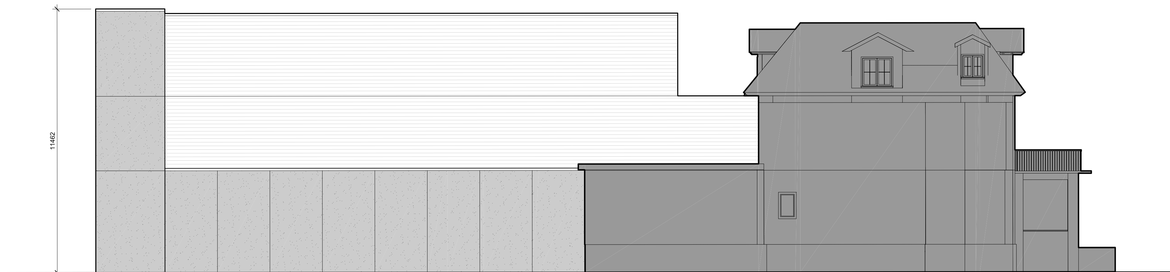
2 A200 WEST ELEVATION 1:100
