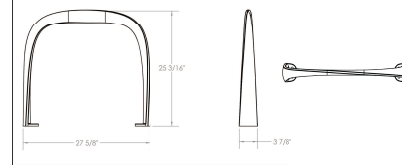
3 BIKE RACK N.T.S.
