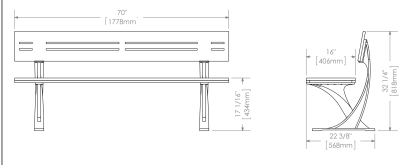
2 BENCH N.T.S.
