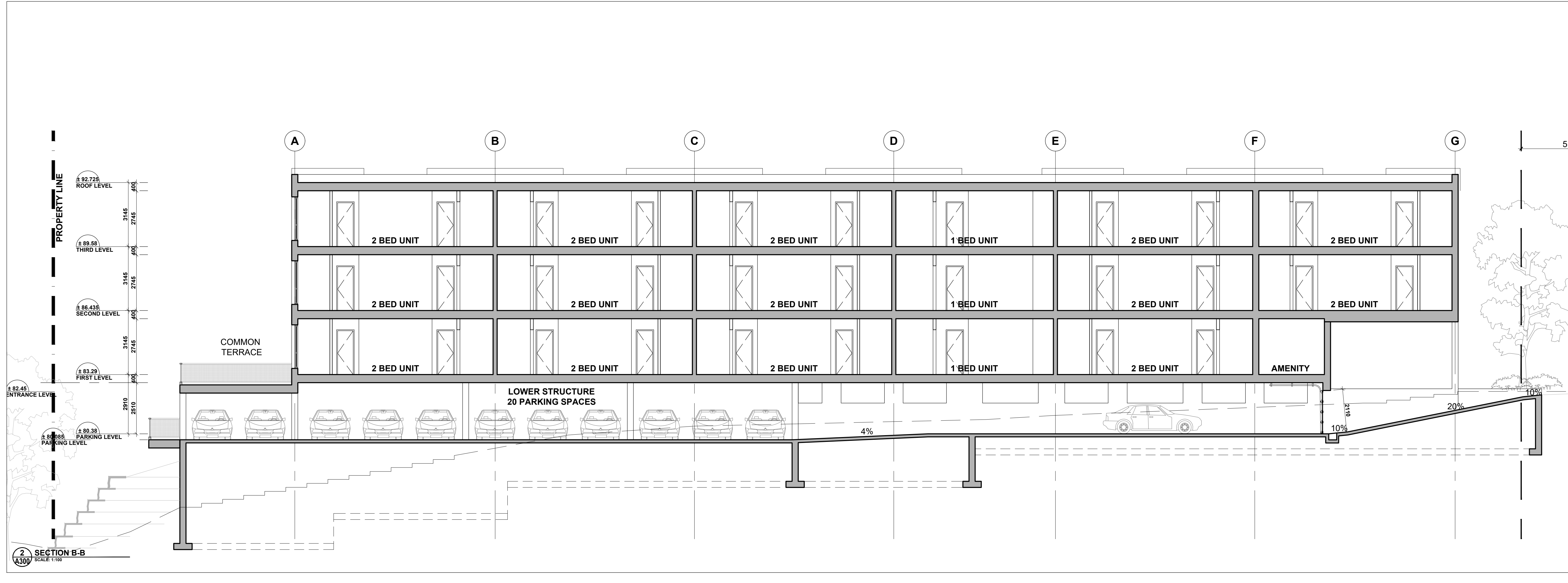
SECTION A-A SCALE: 1:100
