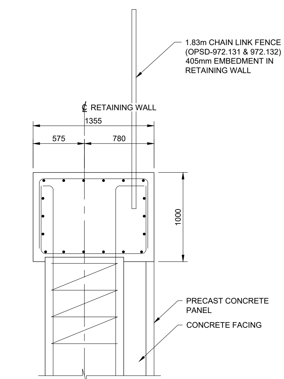
SECTION 2 1:25
