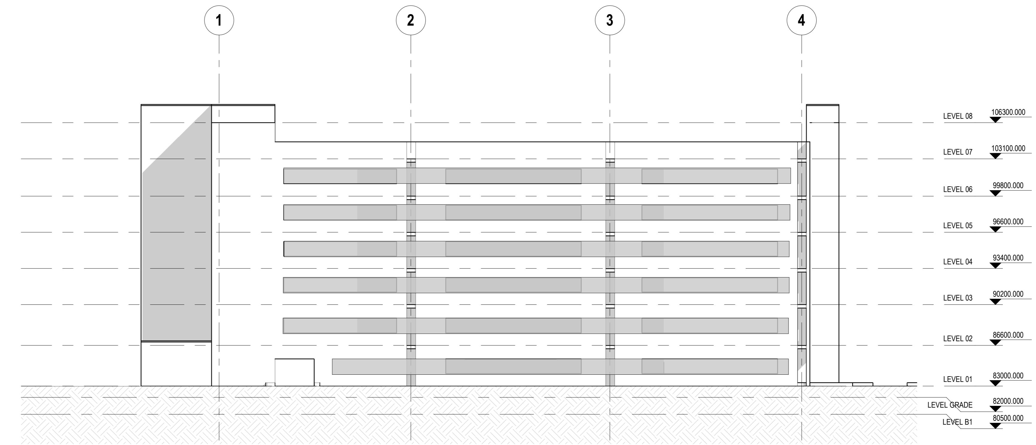
4 ELEVATION 1:200
