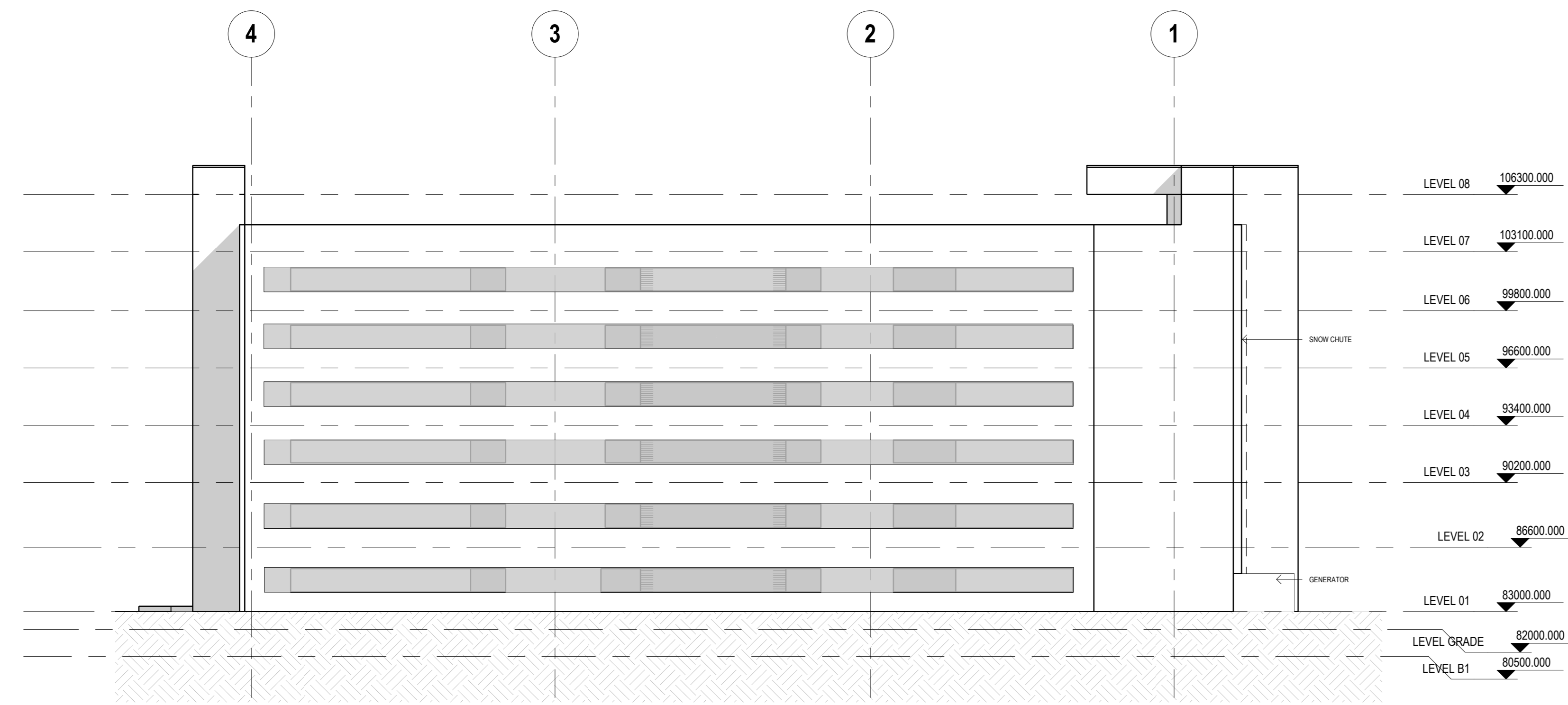
3 ELEVATION 1:200
