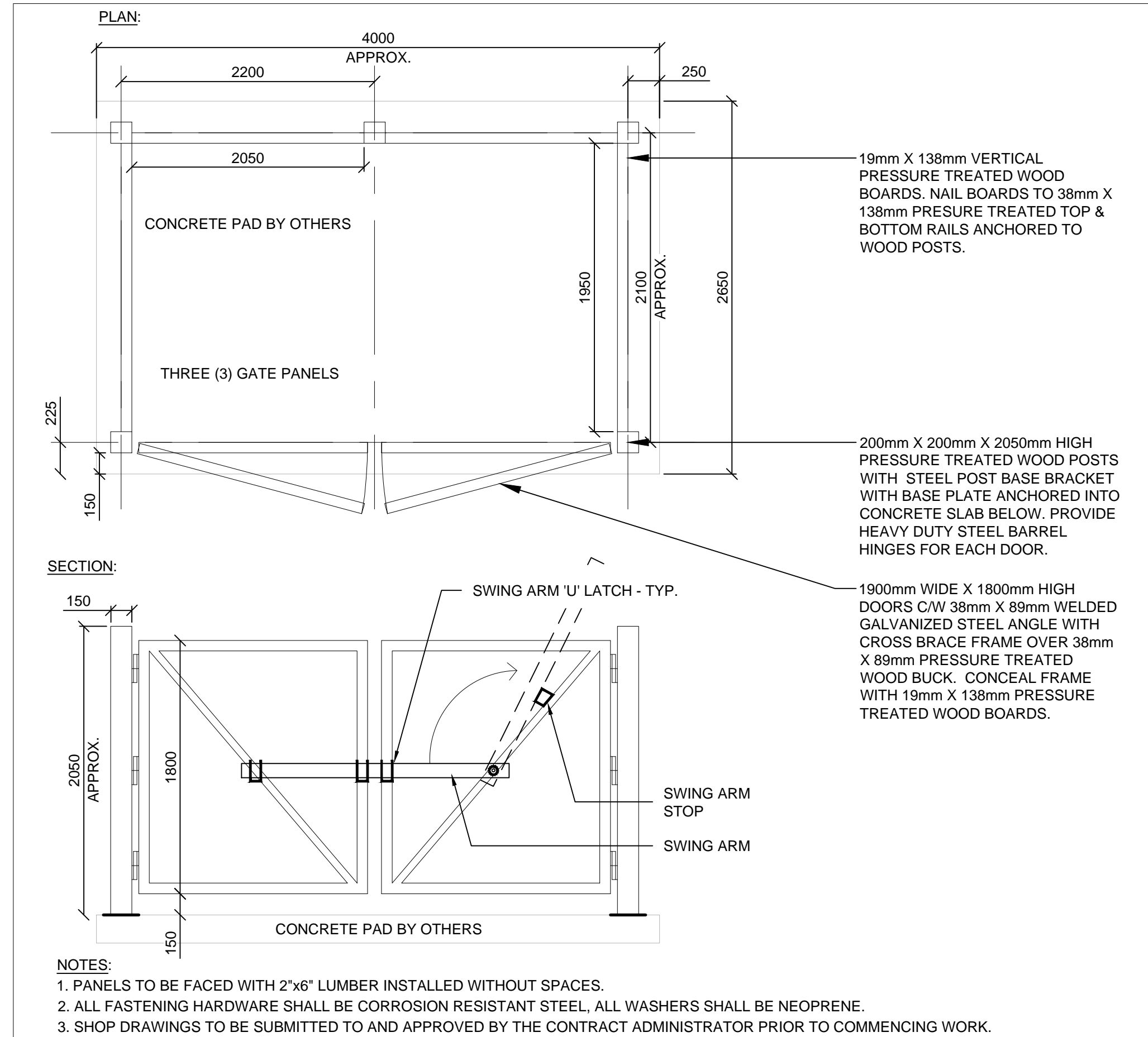
3 GARBAGE ENCLOSURE Scale: 1:30
