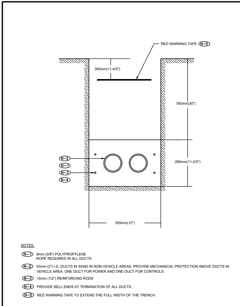
1 E100 LIGHT DUCTS - DIRECT BURIED SCALE: N.T.S.
