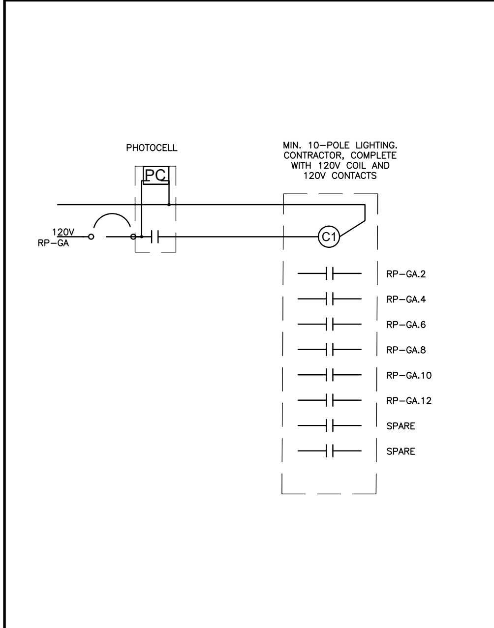
1 E100 EXTERIOR LIGHTING CONTROLS SCHEMATIC SCALE: N.T.S.
