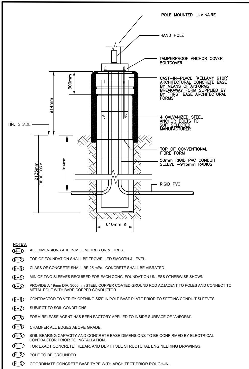
1 E100 LIGHT STANDARD BASE DETAIL SCALE: N.T.S.
