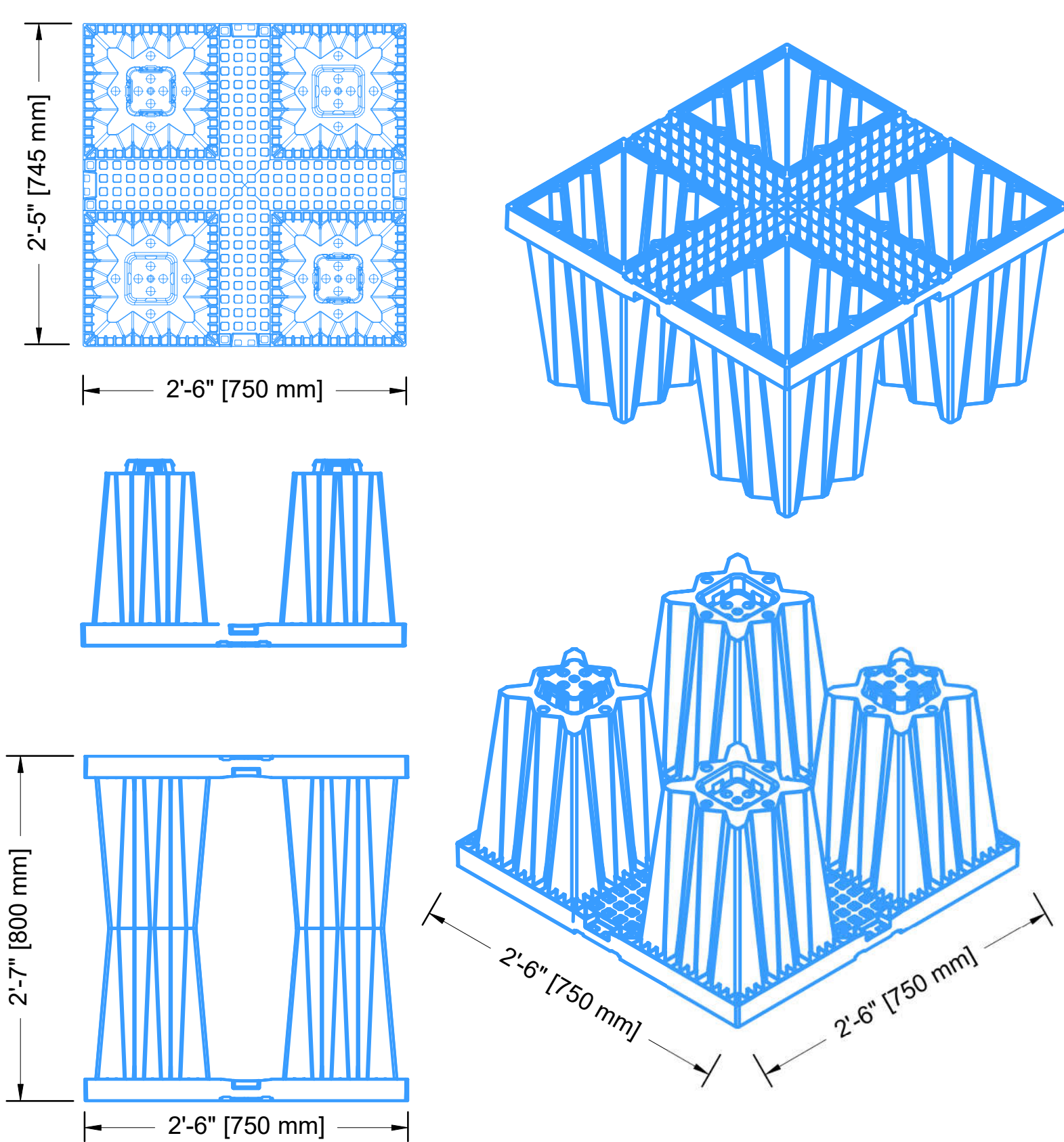
1 AQUABOX HP S-03
