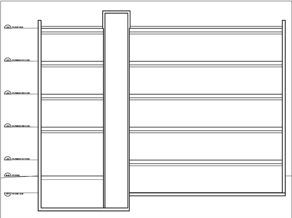
6 LONGITUDINAL SECTION A2 SCALE = 1/16" = 1'-0"
