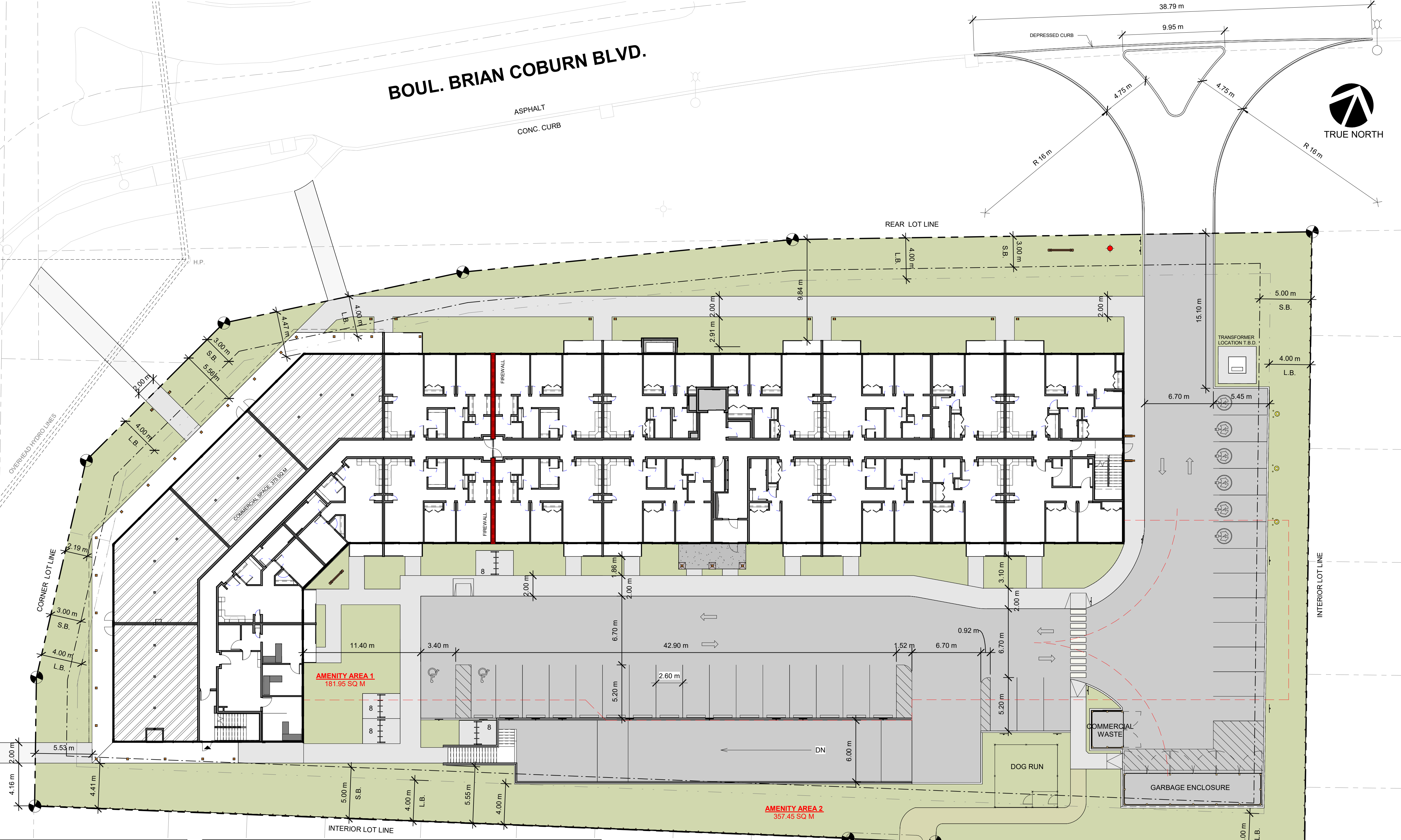
1 SITE PLAN 1:200
