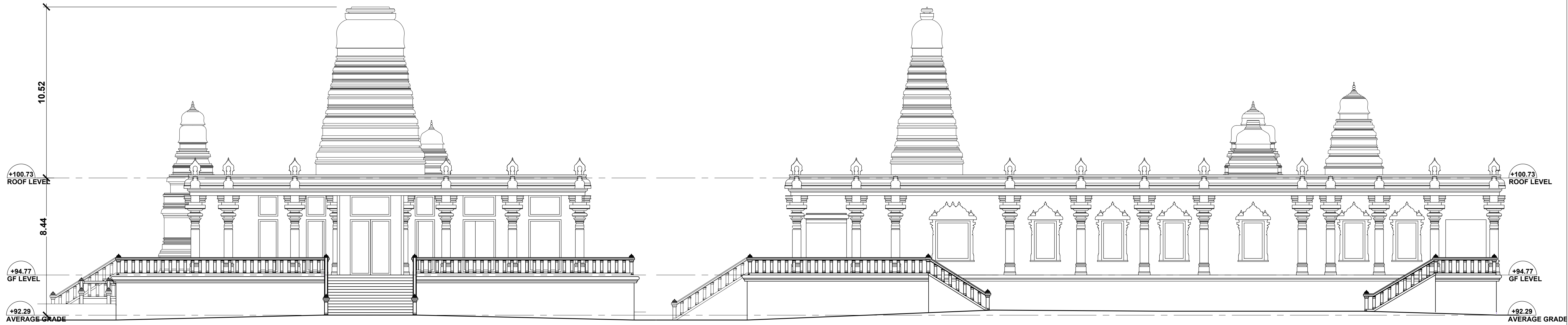
1 EAST ELEVATION SCALE: 1/75
