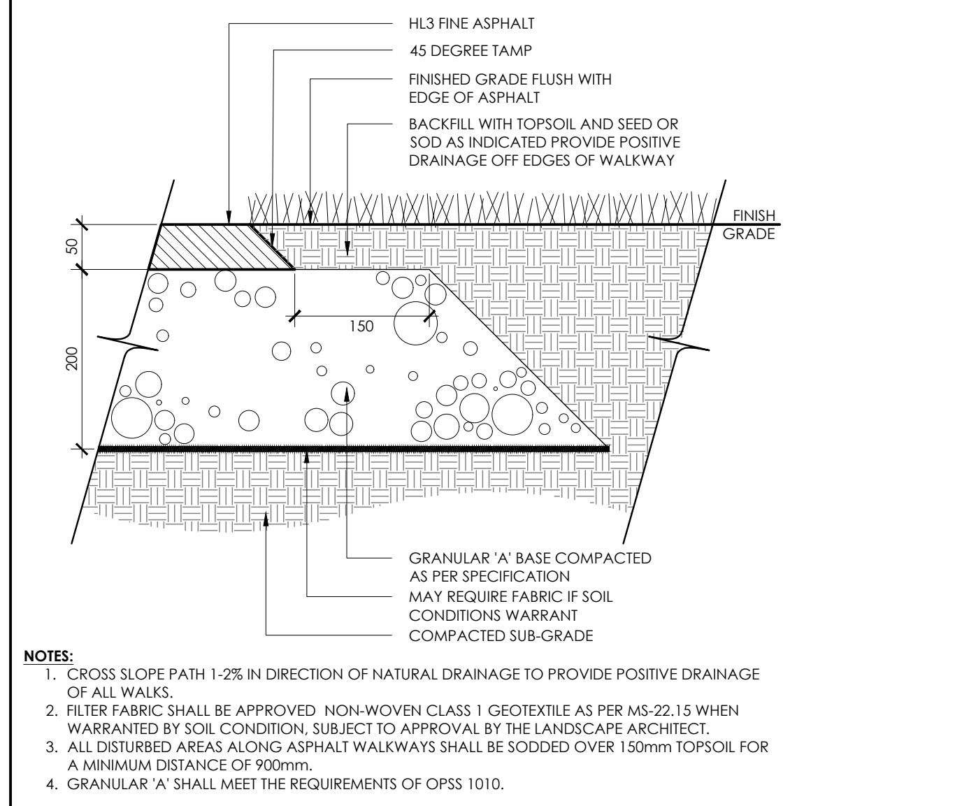
9 LIGHT DUTY ASPHALT PAVING N.T.S.
