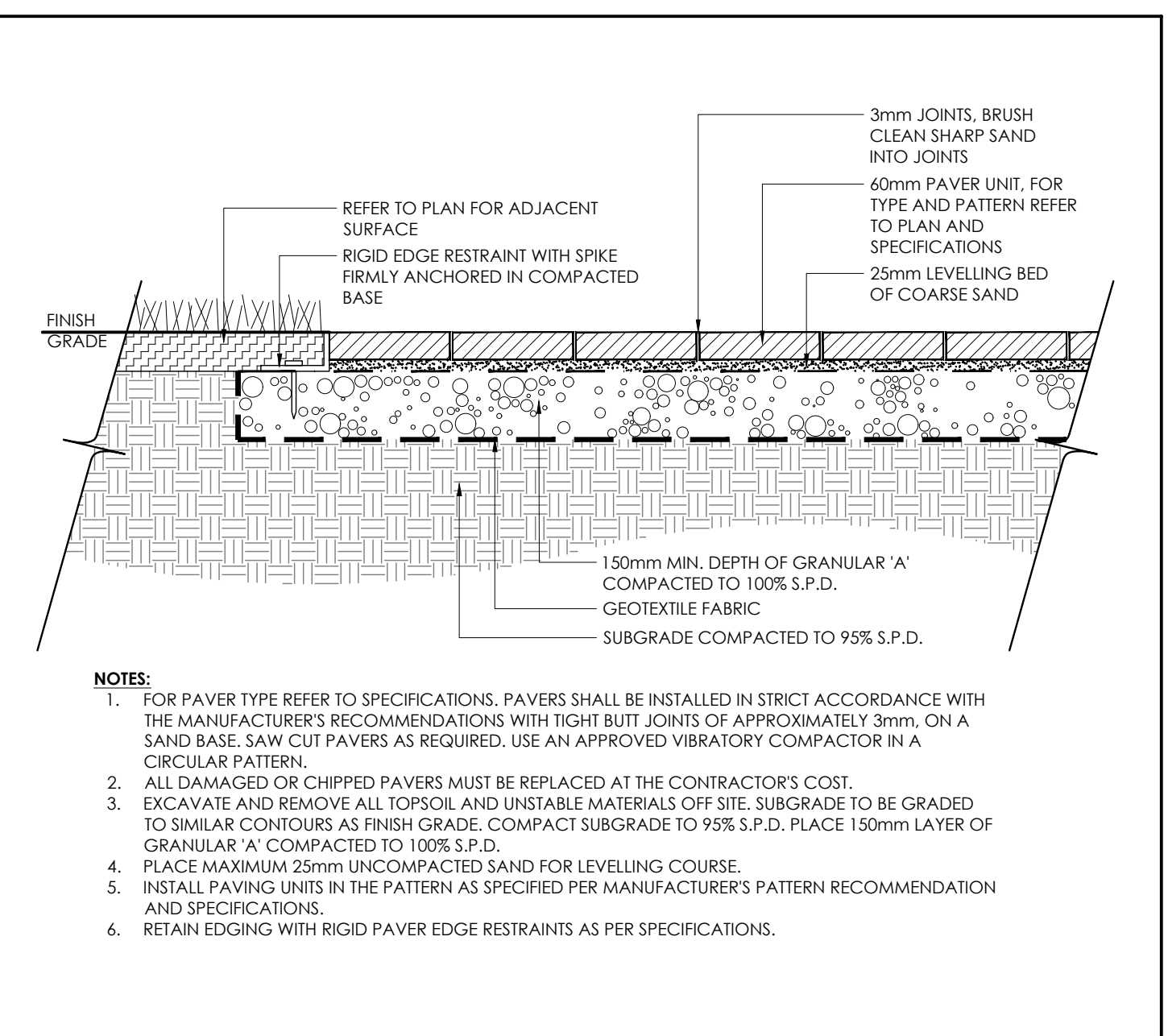
4 LIGHT DUTY UNIT PAVING N.T.S.
