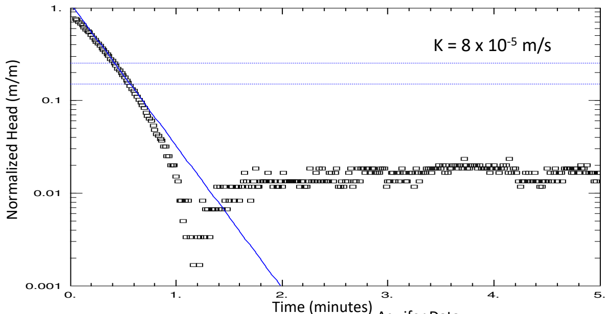
Borehole 21-01 FH: Hvorslev Analysis
