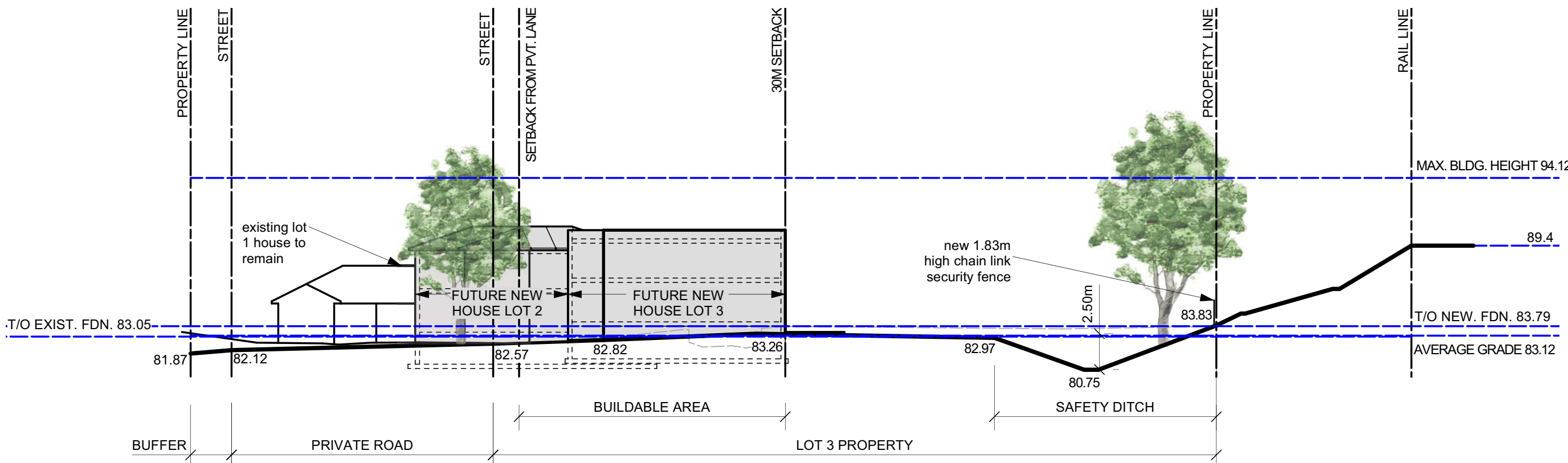
SITE SECTION 1-1 scale: 1:300
